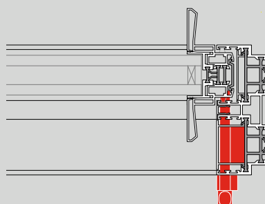
sliding | one point | frame coulissante | un point | cadre
