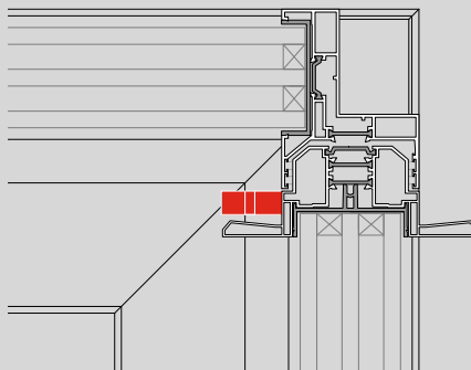
sliding | multipoint | corner coulissante | serrure multipoint | ouverture d'angle
