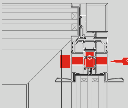
sliding | two points, shootbolt | corner coulissante | deux point | ouverture d'angle
